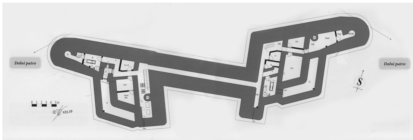
Pevnost MO-S 5 v Bohumíně – řez dolním patrem. Zdroj: Klub vojenské historie Bohumín
